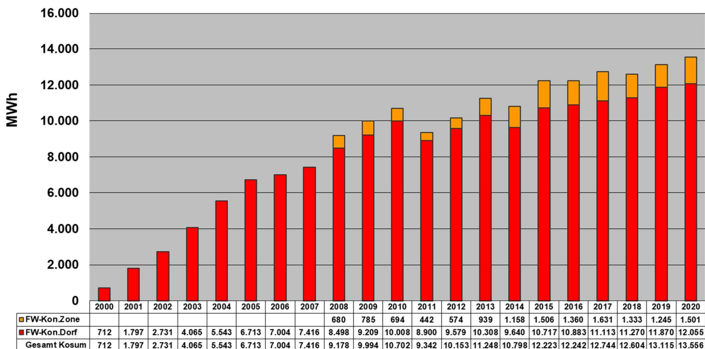
EWP Fernwärmekonsum historisch
