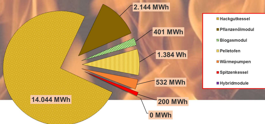
EWP Fernwärmekonsum historisch
